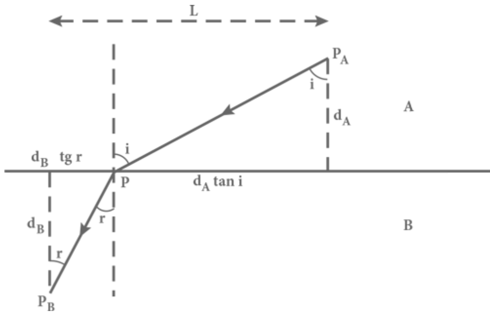
Рис. 21. Путь луча света, испытывающего преломление. Горизонтальной линией отмечена граница двух прозрачных сред A и B , в которых свет имеет различные скорости v_A и v_B . Углы i и r измеряются между направлениями светового луча и вертикальной штриховой линией, обозначающей перпендикуляр к границе раздела сред. Сплошная линия со стрелками отмечает путь следования луча из точки PA в среде A до точки P на границе раздела сред и затем до точки PB в толще среды B .
