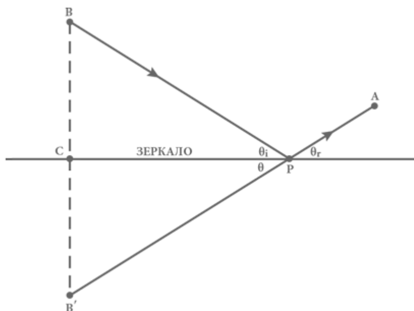
Рис. 3. Доказательство теоремы Гермона. Теорема доказывает, что кратчайший путь из объекта B до поверхности зеркала и затем к наблюдателю в точке A таков, что углы \theta_i и \theta_r равны. Начерченные сплошной линией отрезки помечены стрелками, показывающими
