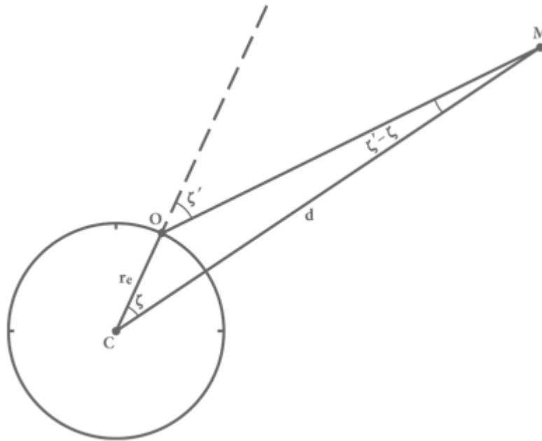
Рис. 8. Использование параллакса для определения расстояния до Луны. Здесь \zeta' – угол между наблюдаемым положением Луны и вертикалью, а \zeta – то значение, которое было бы у этого угла, если можно было наблюдать Луну из центра Земли.
